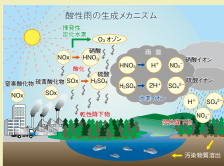
図2 酸性雨の生成メカニズム *3)
