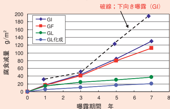
図-3 めっき材の腐食減量（上向き曝露）
