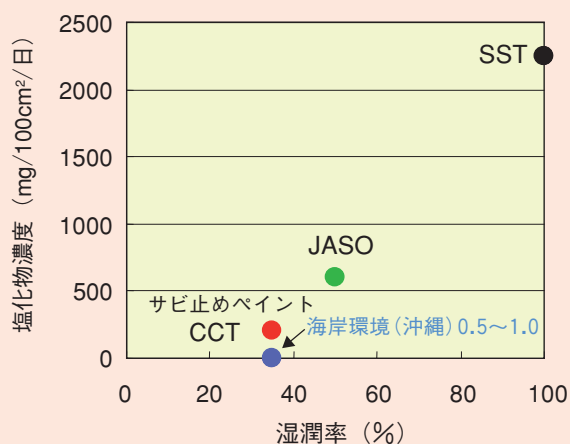
図-9 各促進試験と塩化物濃度、湿潤率の関係
