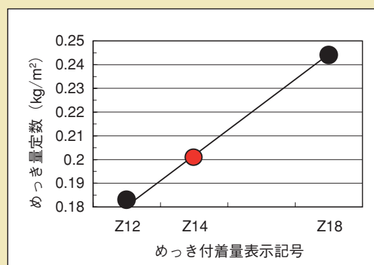
図-2 Z14のめっき量定数
