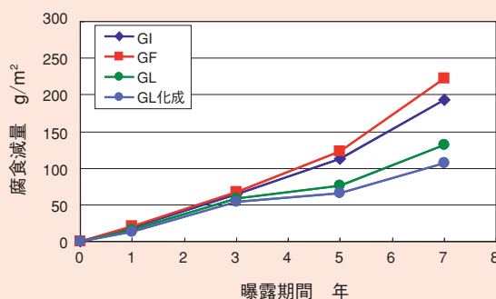
図-4 めっき装材の腐食減量（下向き曝露）
