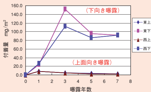
図-5 塩素イオン付着量；GIめっき
