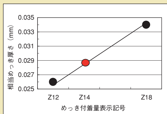
図-1 Z14の相当めっき厚さ
