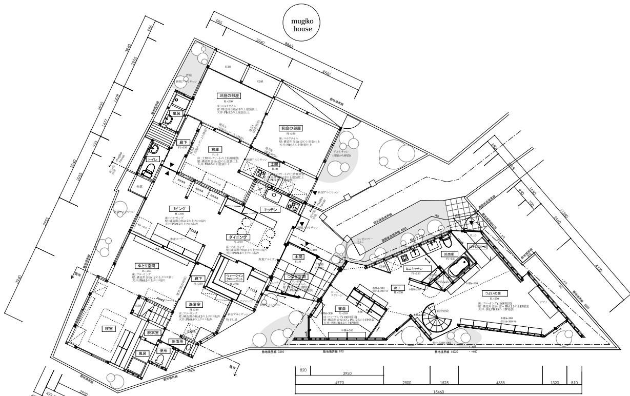
2 階平面図
