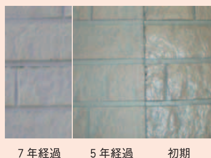
窯業系サイディング 上向き曝露試験結果
