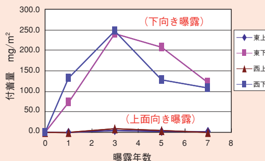
図-7 硫酸イオン付着量；GIめっき
