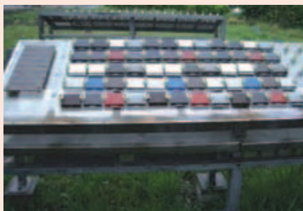
曲げ加工サンプルの曝露状況
