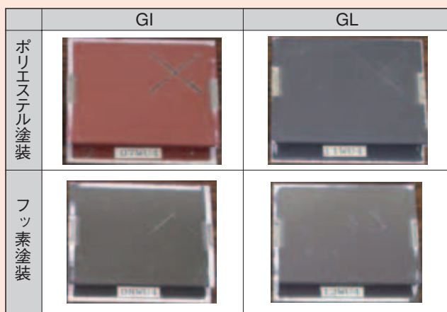
図-8 塗装材 上向き曝露試験結果
